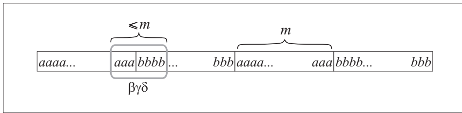
Rys. 4.8: Ilustracja do Przykładu 4.15. Segment \beta\gamma\delta ze względu na ograniczoną długość nie większą niż m może mieścić się w obrębie co najwyżej dwóch sąsiednich bloków liter a i b . W każdym z możliwych położeniach pompowanie niszczy symetrię słów języka L .
