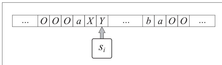
Rys. 6.1: Klasyczna jednotaśmowa maszyna Turinga.
