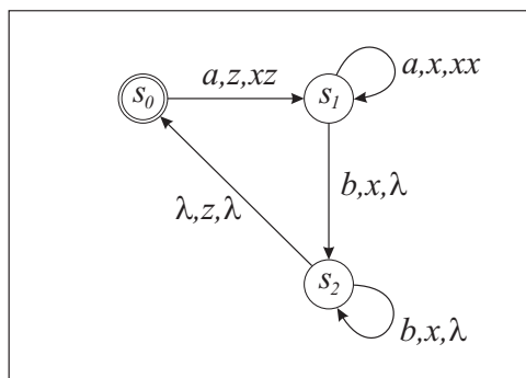
Rys. 4.5: Deterministyczny automat ze stosem akceptujący język \{a^n b^n : n \geq 0\} z Przykładu 4.8.
