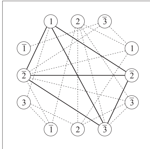
Rys. 7.2: Graf dla formuły \Phi danej w równaniu (7.1). Wierzchołek oznaczony symbolem 1 odpowiada zmiennej x_1 , symbolem \bar{2} — zmiennej \bar{x}_2 itd. Dla czytelności rysunku pominęliśmy niektóre krawędzie.
