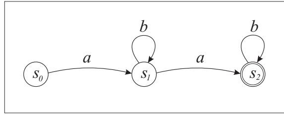
Rys. 3.2: SAD akceptujący język z Przykładu 3.1.
