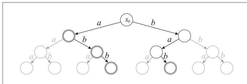
Rys. 3.5: Automat w postaci drzewa dla skończonego języka L = \{a, ab, abb, bab\} . Szarym kolorem oznaczyliśmy krawędzie i stany, które mogą być usunięte z ostatecznej wersji grafu.
