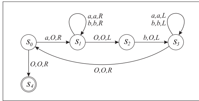
Rys. 6.2: Maszyna Turinga akceptująca język L = \{a^n b^n : n \geq 0\} , Przykład 6.1.
