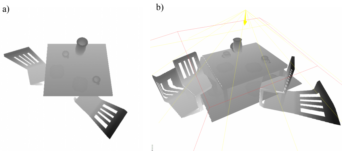
Rys. 20. Mapa cieni a) utworzona przy pomocy kamery ustawionej w punkcie źródła światła oraz b) jej projekcja na geometrię sceny.
