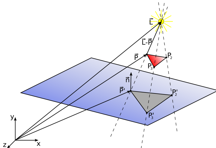
Rys. 3. Tworzenie cienia poprzez rzutowanie perspektywiczne obiektu na płaszczyznę.
