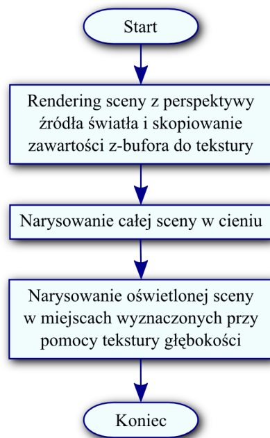
Rys. 19. Diagram przedstawiający trzy przebiegi renderingu wymagane do wykonania obrazu przy pomocy metody mapowania cieni.
