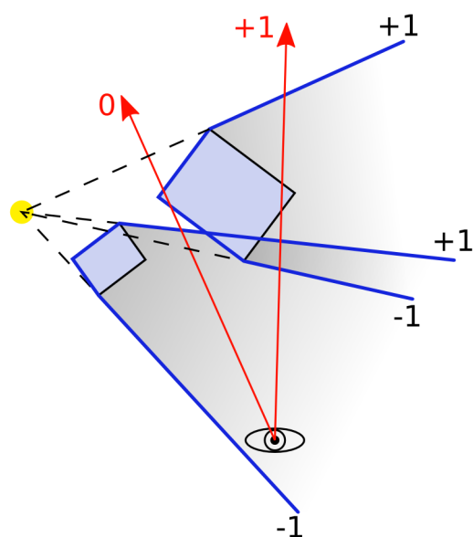
Rys. 15. Ilustracja poprawności działania algorytmu stencil fail ( z-fail ) dla przypadku, w którym obserwator znajduje się wewnątrz cienia.
