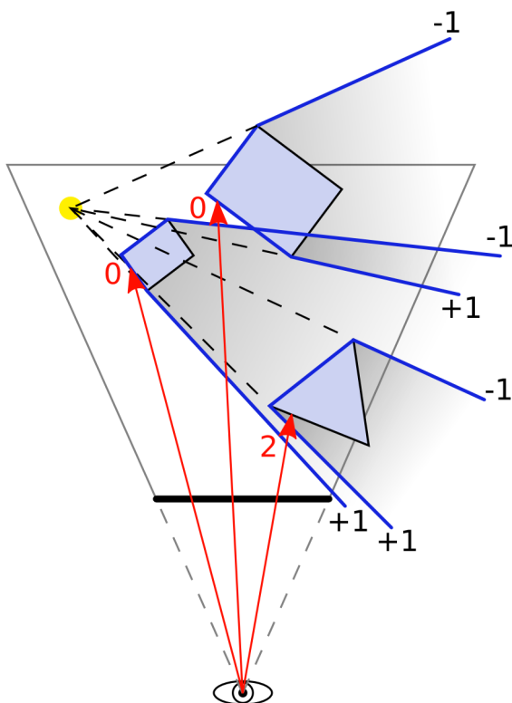
Rys. 12. Działanie algorytmu stencil pass ( z-pass ).
