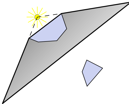
Rys. 11. Skończona bryła cienia powstała poprzez wytłoczenie obrysu obiektu na ustaloną z góry odległość. Na ilustracji widać, że nie pokrywa ona jednego z obiektów sceny.
