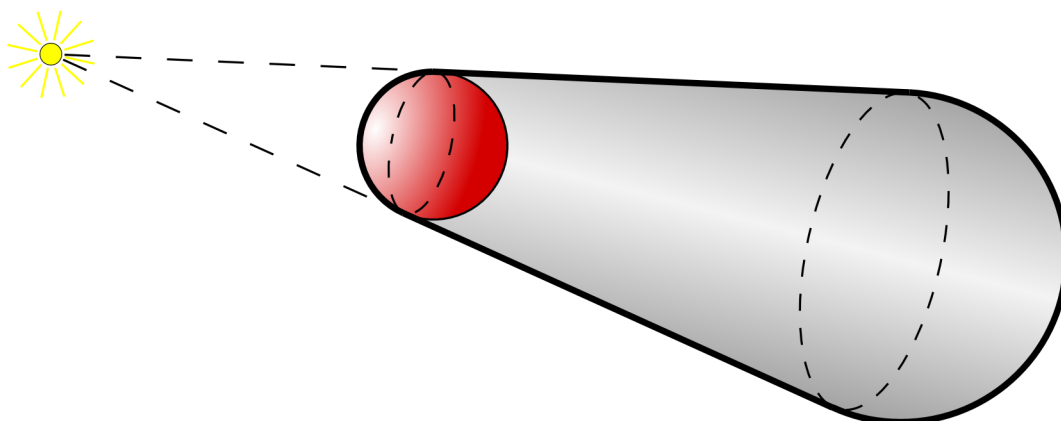
Rys. 8. Bryła cienia dla sfery. Linie przerywane zaznaczają kontury blokującego światło obiektu (z punktu widzenia światła). Pokazują również podział powierzchni bryły na trzy części (odpowiednio od lewej): domknięcie przednie, boki oraz domknięcie tylne.
