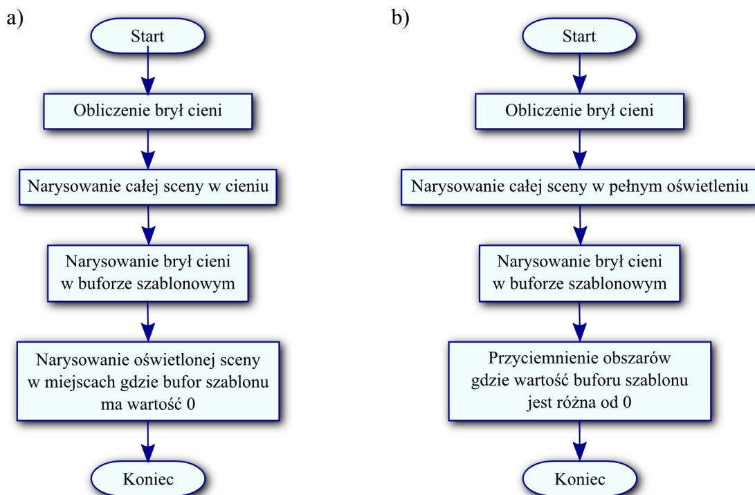
Rys. 7. Algorytm rysowania cieni obiektów a) poprzez dwukrotne rysowanie sceny: w cieniu i w pełnym świetle lub b) poprzez przyciemnianie odpowiednich obszarów znajdujących się w cieniu.
