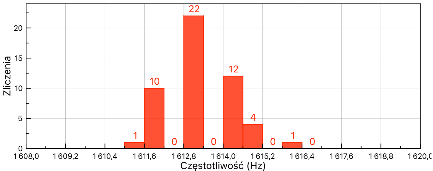
Generator z mostkiem Wiena
